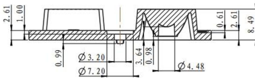
截面 AA-AA
